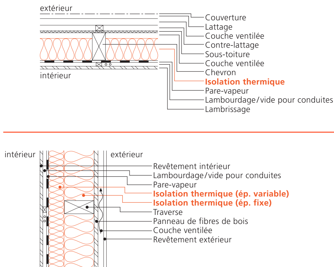
Fig. 5 Exemple d'éléments inhomogènes.
